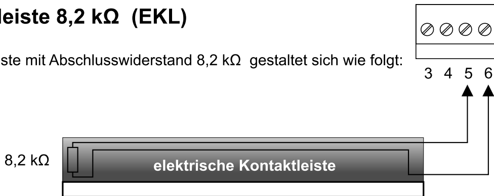
Abb. 5-5, Anschluss elektrische Kontaktleiste 8,2kΩ
