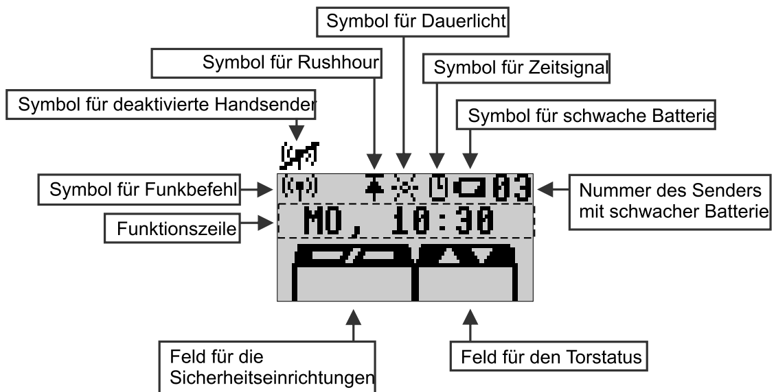
Abb. 4-2, Anzeigeelemente
