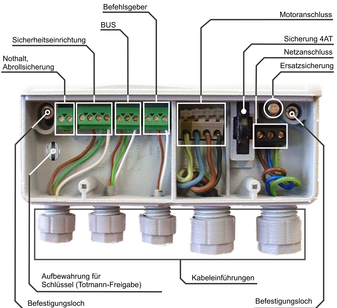
Abb. 5-2, Klemmenbereich
