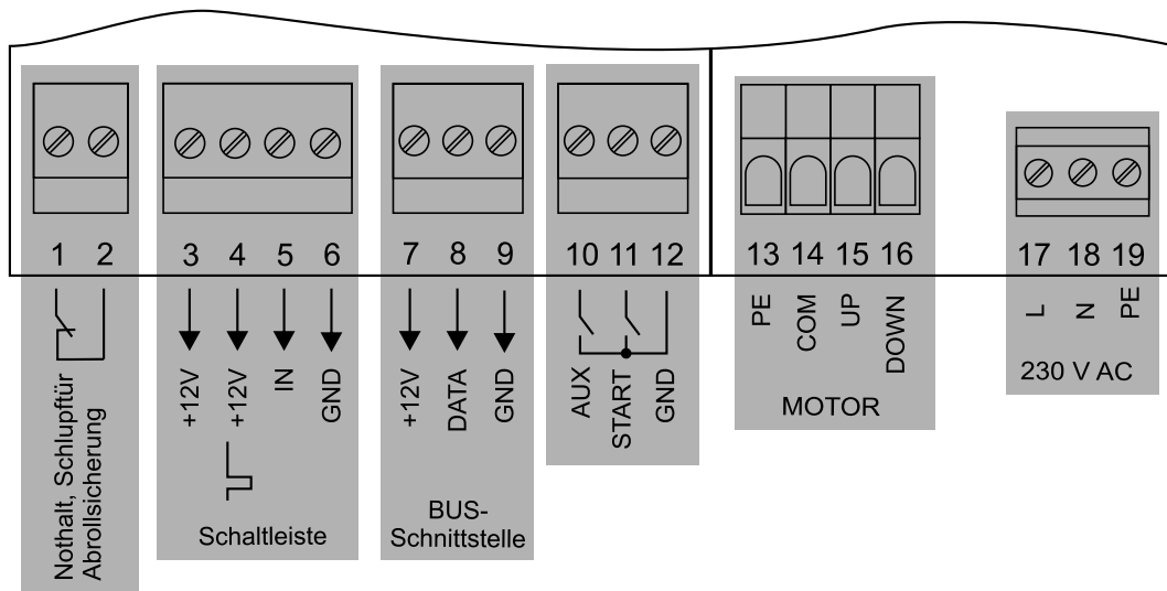
Abb. 5-3, Anschlussplan
