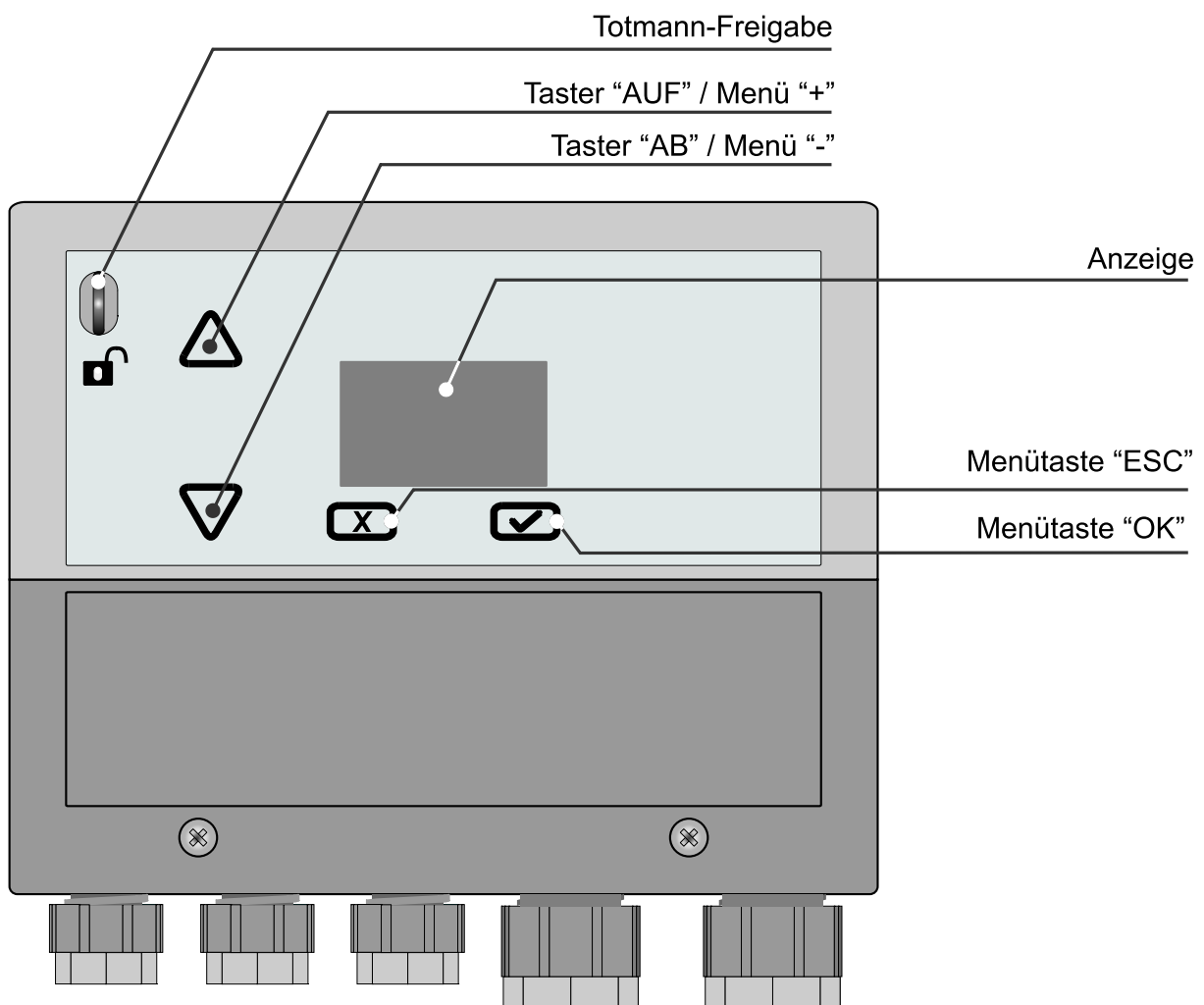
Abb. 4-1, Bedien- und Anzeigeelemente
