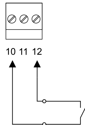
Abb. 5-11, Anschluss Vorendlagenschalter
