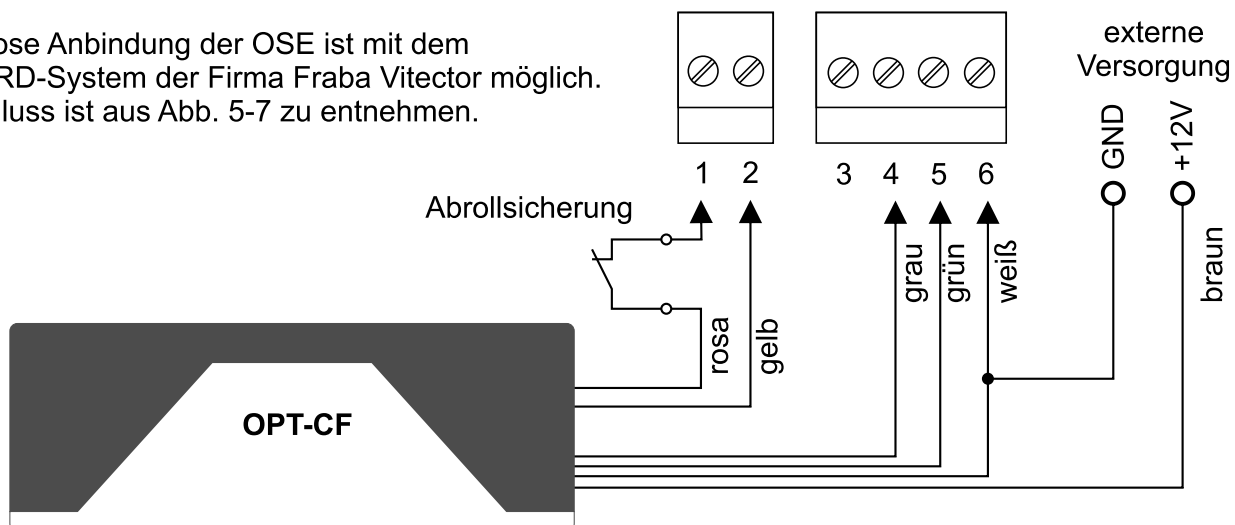
Abb. 5-7, Anschluss OPTOCORD
