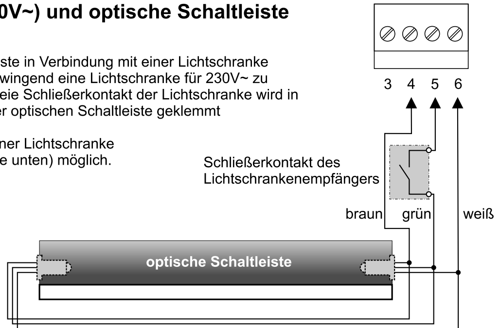
Abb. 5-10, Anschluss Lichtschranke (230V~) und OSE
